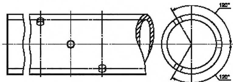
Рисунок Г.1 — Эталонный образец с тремя отверстиями
