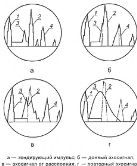
Рисунок В.1 — Вид эхосигналов на экране дефектоскопа
